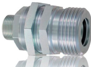
Rohrleitungskupplung-Muffe Typ RK-DN...-M / Screw on couplings fe male type RK-DN...-M Festhälfte; Material: Stahl verzinkt; Dichtung: NBR
